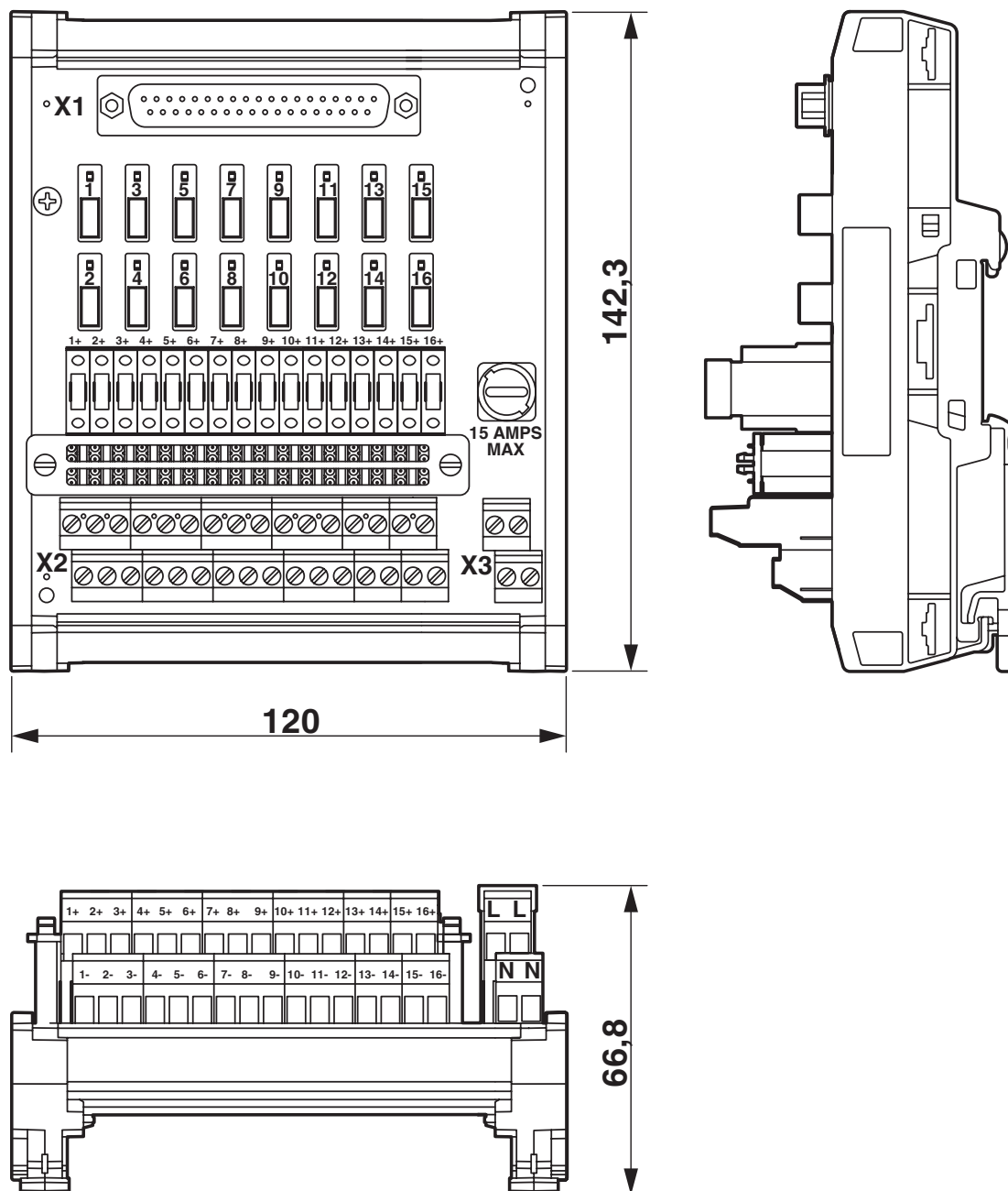
Maßzeichnung
