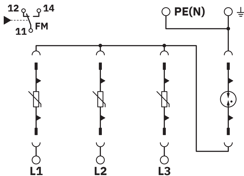
Diagrama eléctrico
