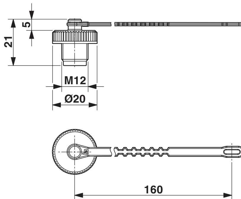
Dessin coté
