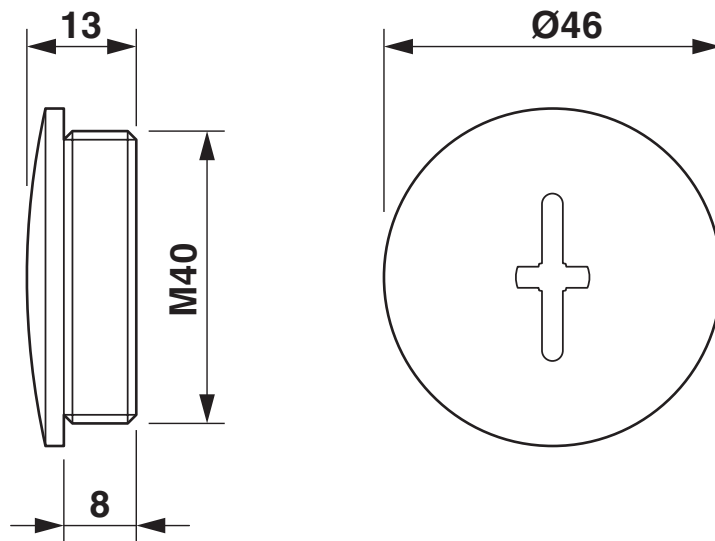
Dessin coté
