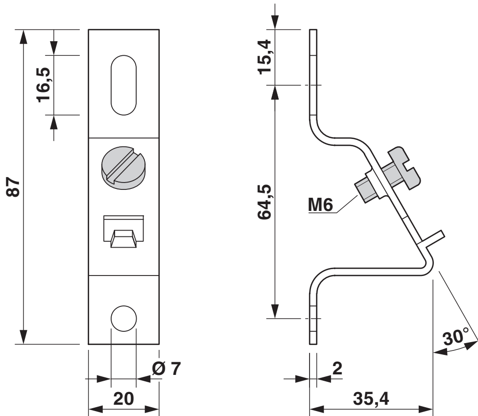
Maßzeichnung
