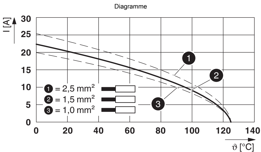
Diagramme de déclassement pour les conducteurs rigides
