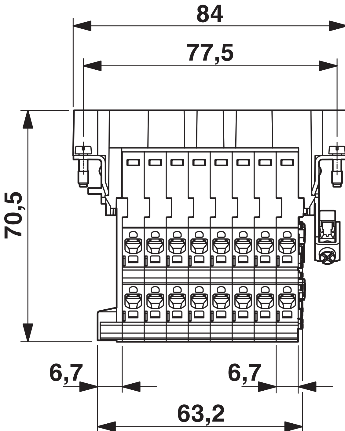
Dessin coté
