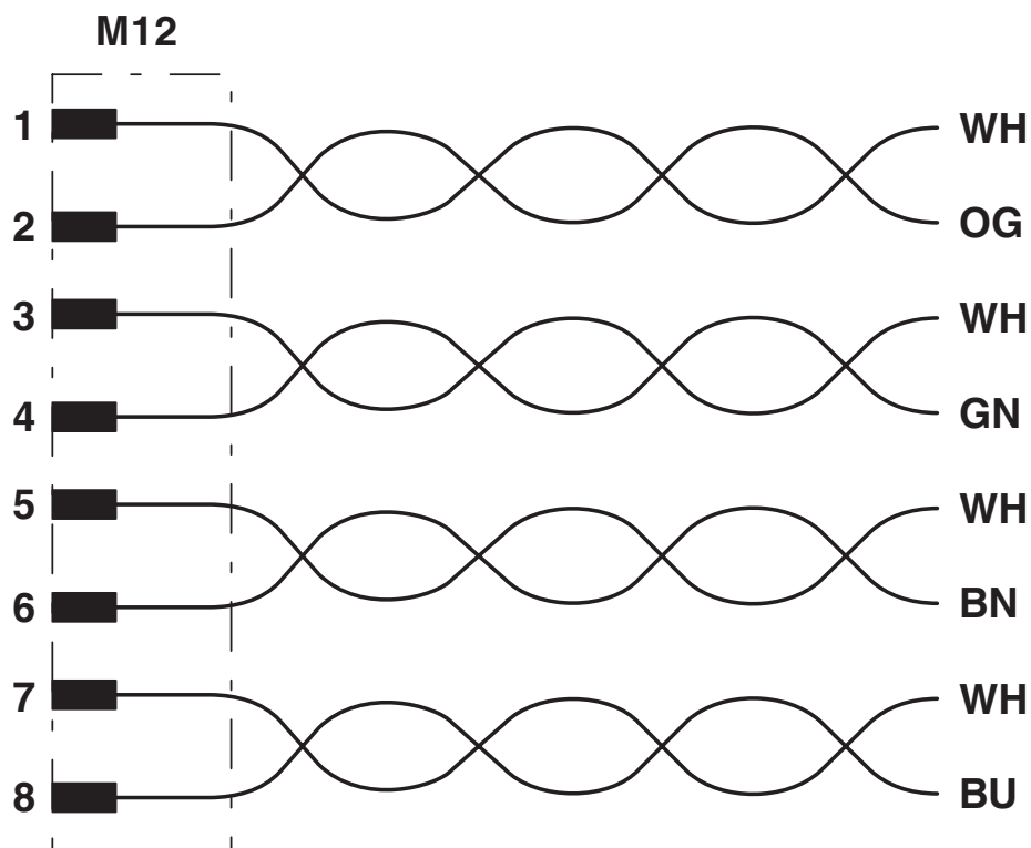
Diagrama eléctrico
