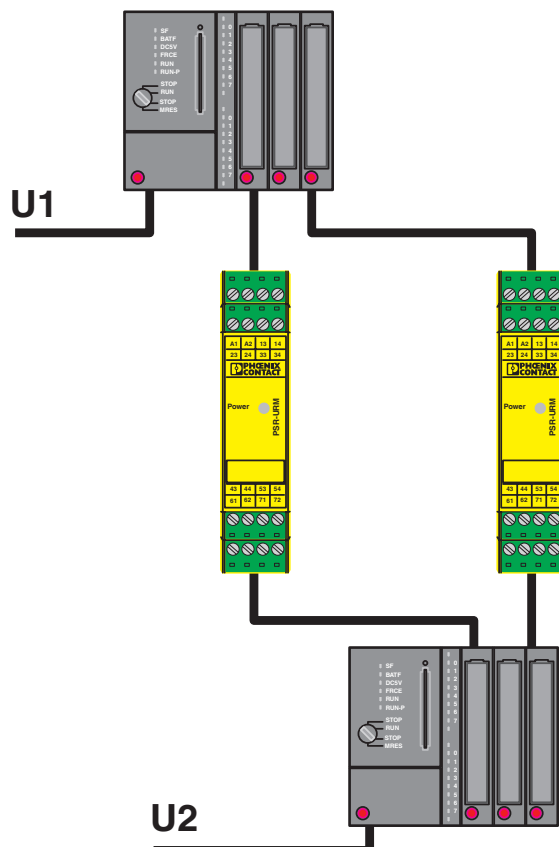
Applikationszeichnung
