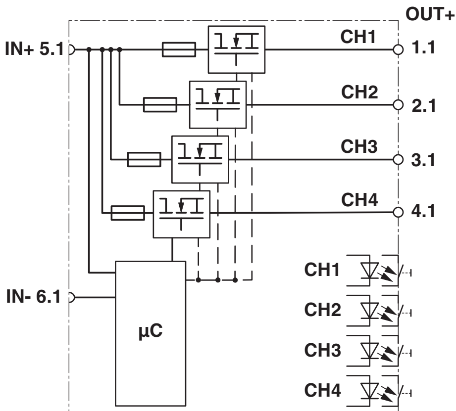
Schéma fonctionnel
