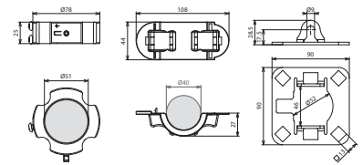
Maßbild BFS SR D40 4AE HVI LI PL AL V2A
