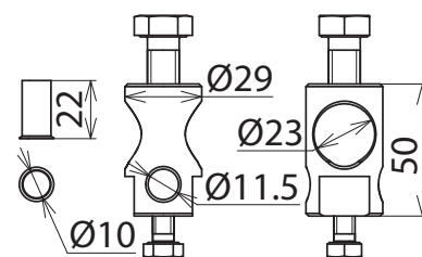
Maßbild BB 1XB11GSM8 1XB23GSM12 AL
