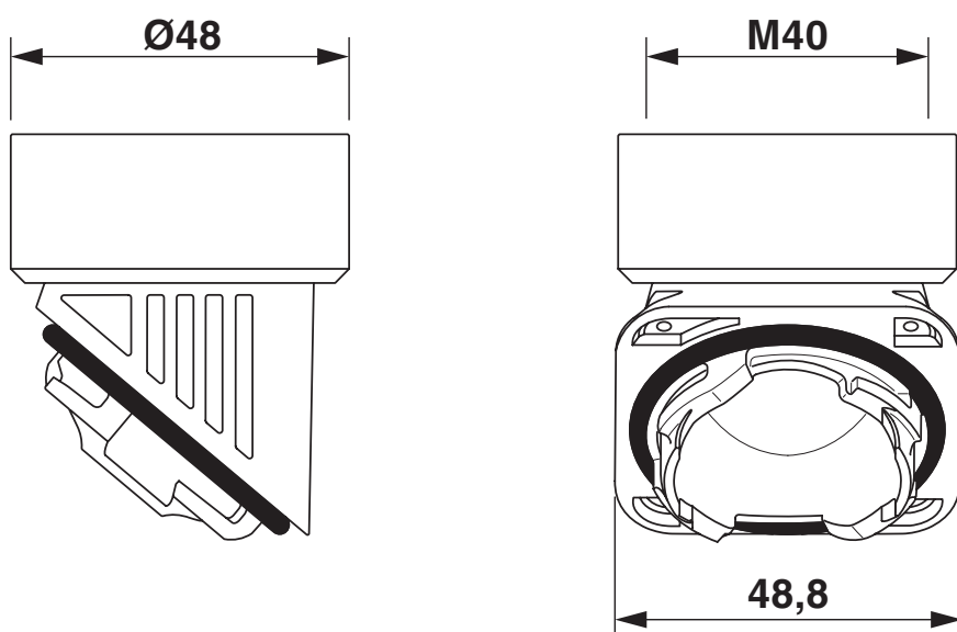
Dessin coté
