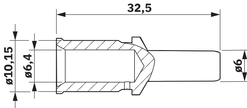
Esquema de dimensiones
