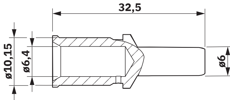
Dessin coté
