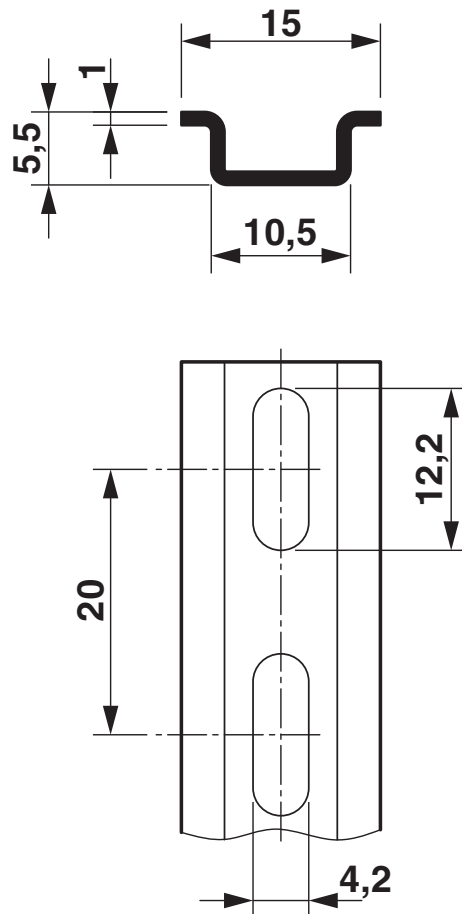
Maßzeichnung
