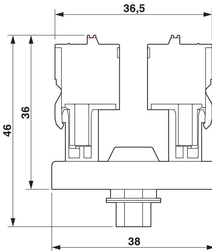
Maßzeichnung
