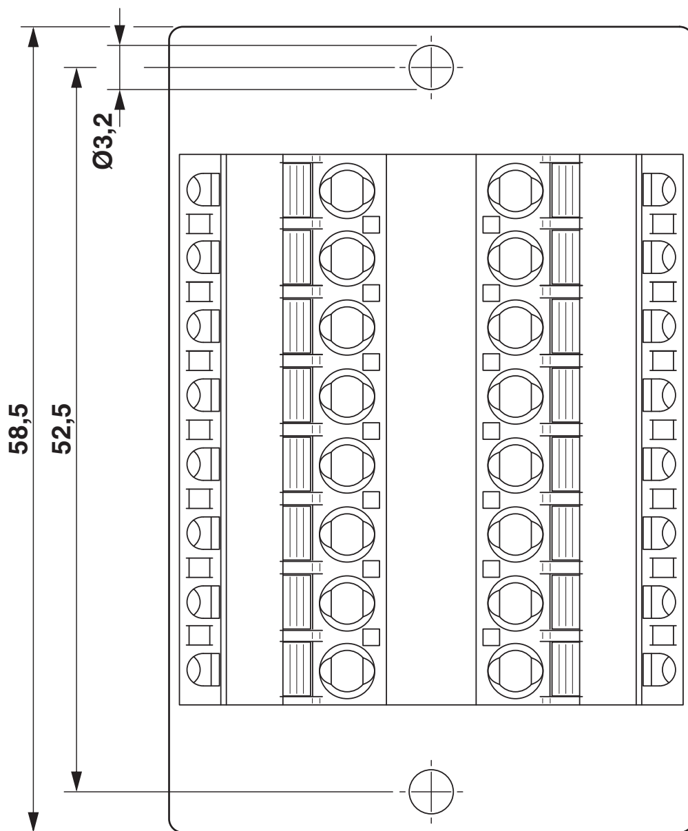
Maßzeichnung
