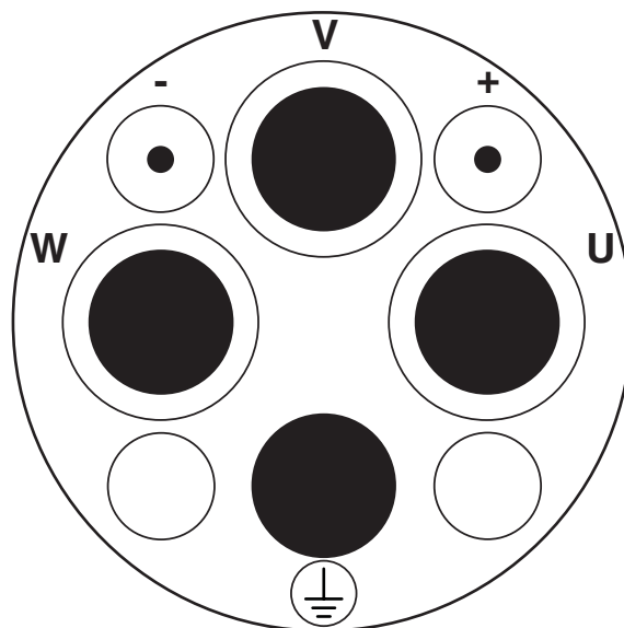
Schemazeichnung
