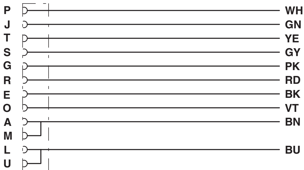
Schaltplan
