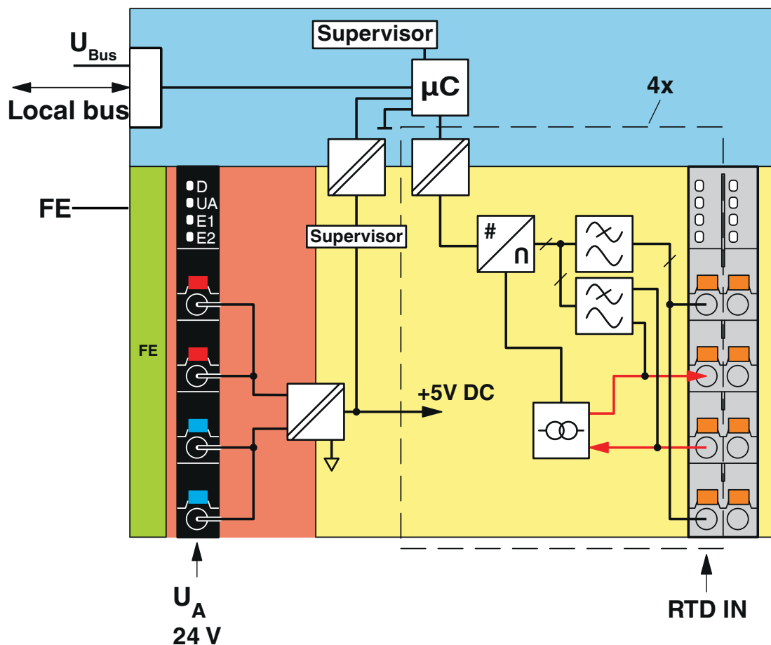
Schéma fonctionnel
