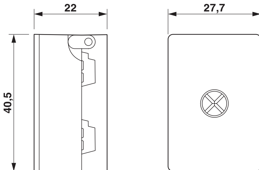
Maßzeichnung
