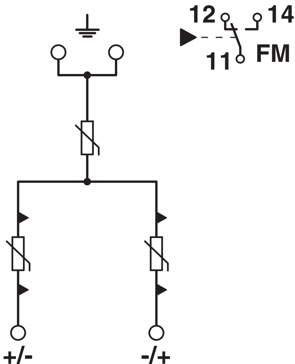
Schaltplan
