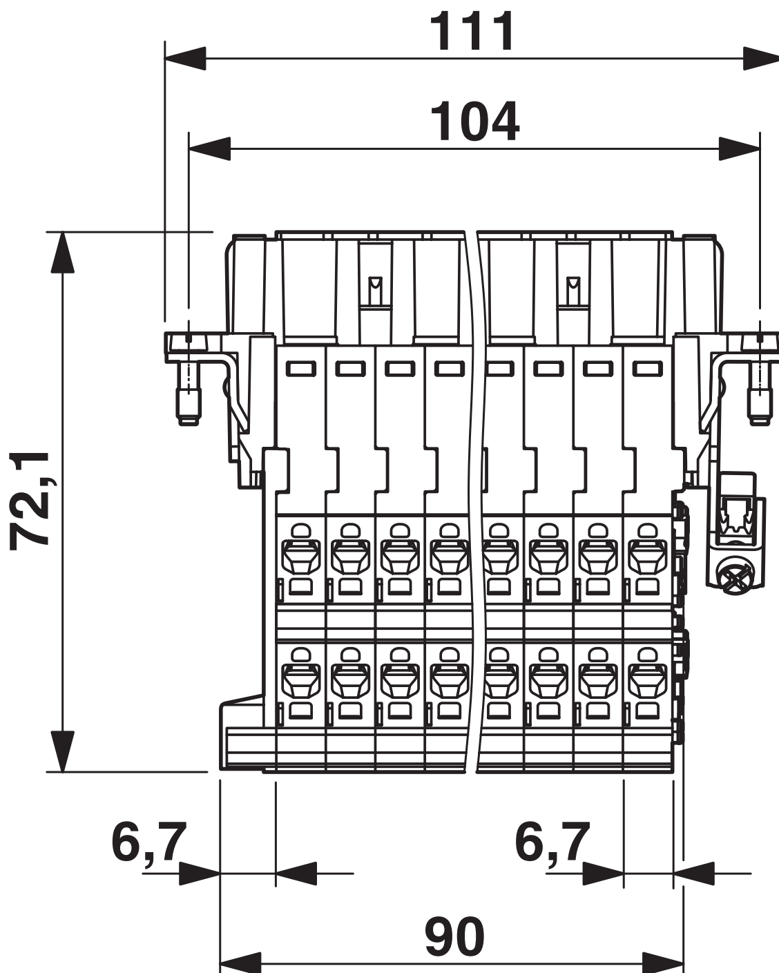
Maßzeichnung
