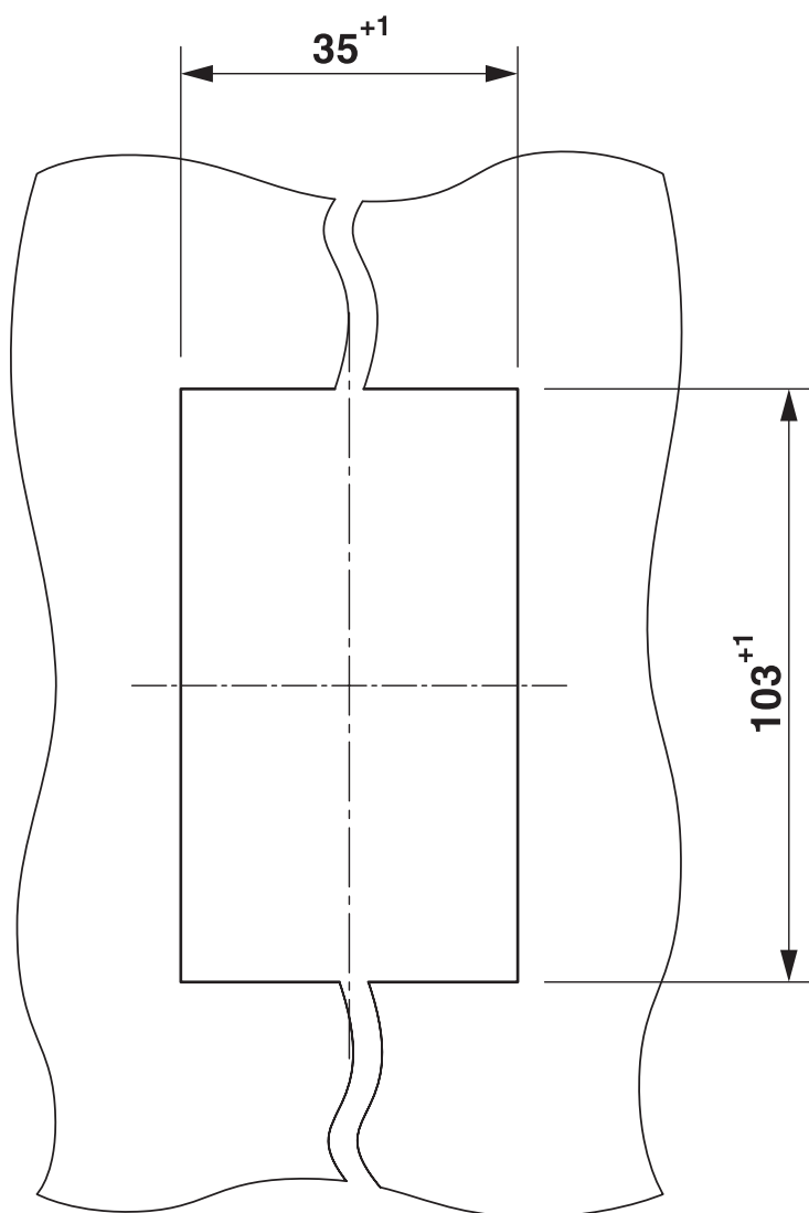
Dessin coté
