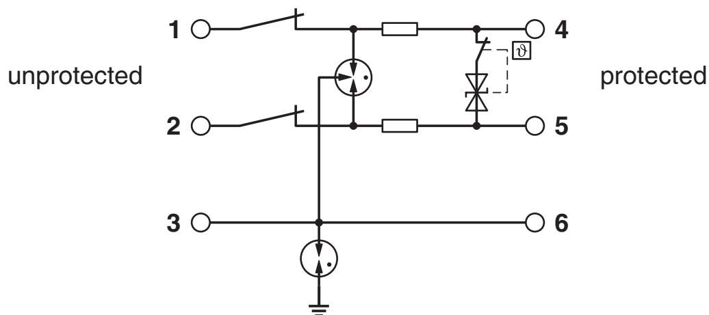
Diagrama eléctrico
