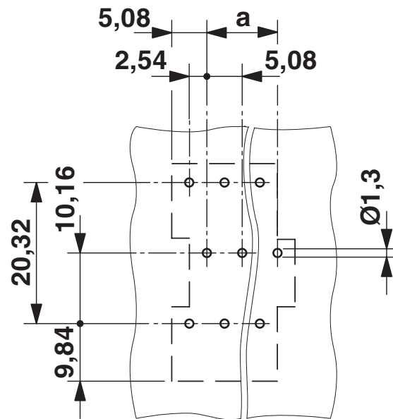
Bohrplan/Lötpadgeometrie
