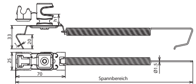
Maßbild DLH SSL 8 H36 FG180.280 GR V2A
