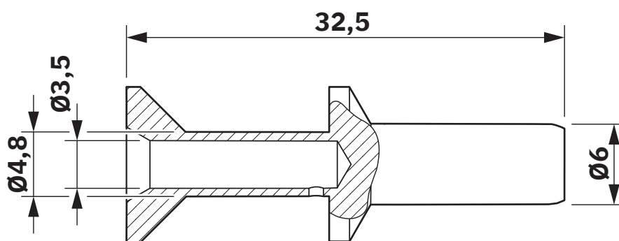
Dessin coté
