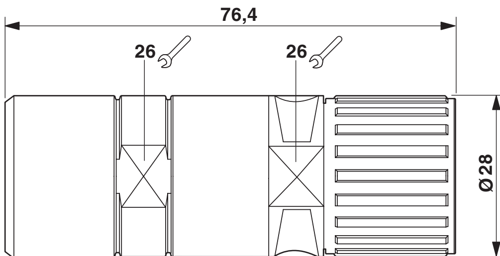
Dessin coté
