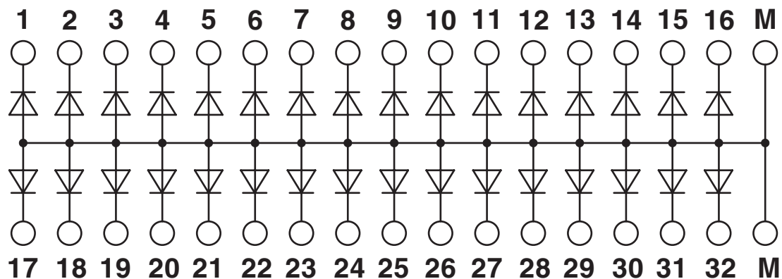
Diagrama eléctrico
