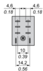
Stecker-Seitenansicht
