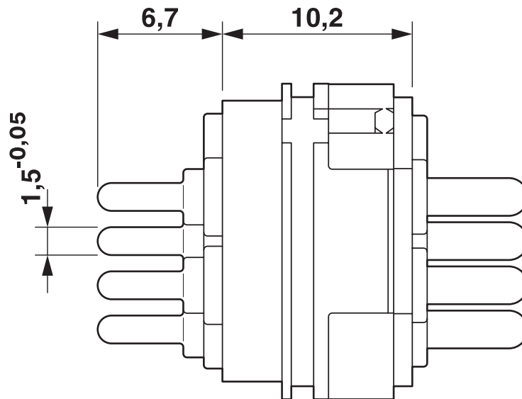
Maßzeichnung
