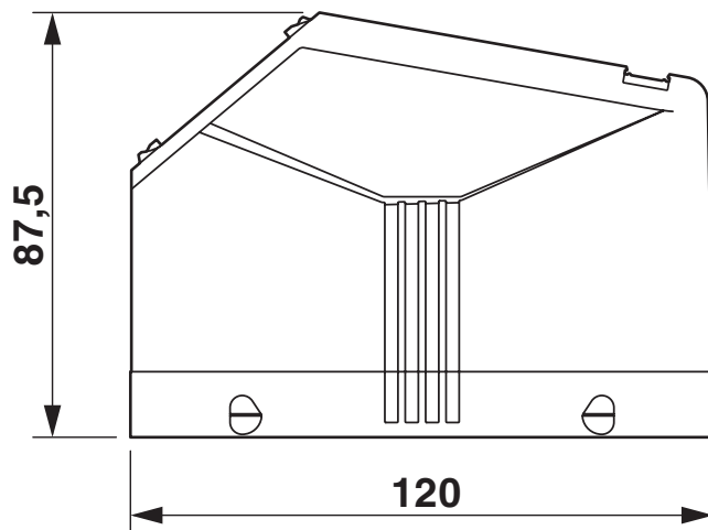
Maßzeichnung
