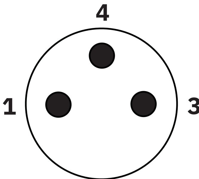
Esquema polos con. macho M8, 3 polos, vista cara machos
