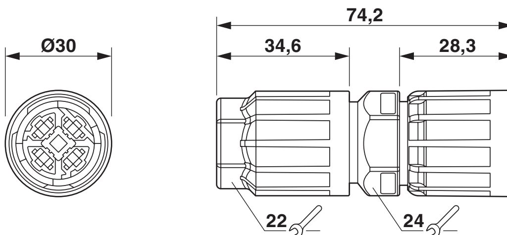
Maßzeichnung
