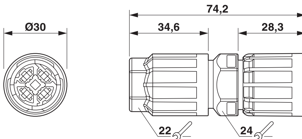
Dessin coté
