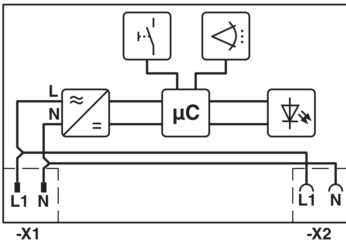
Schéma fonctionnel
