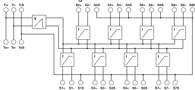
Diagrama eléctrico
