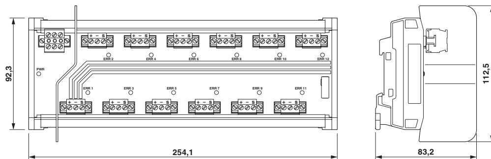
Dessin coté
