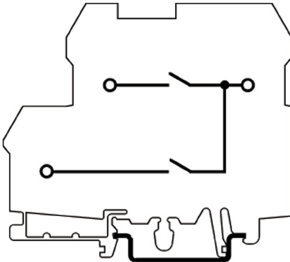
Diagrama eléctrico
