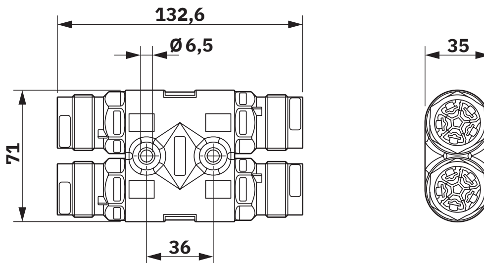
Maßzeichnung
