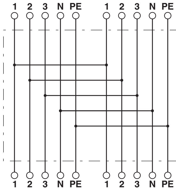
Diagrama eléctrico
