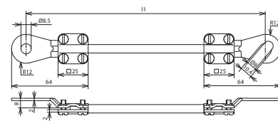
Maßbild EL10 L3.05M 1KSO 8.10 1KSG 8
