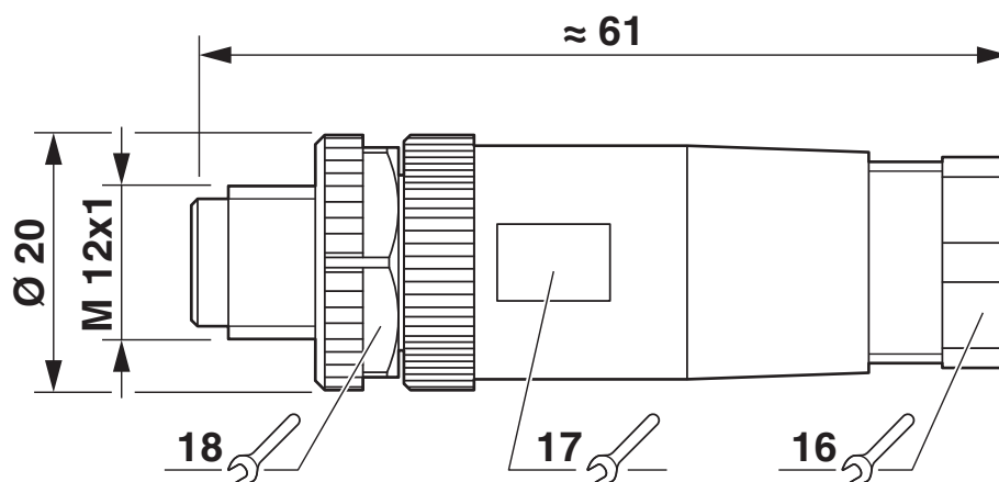
Maßzeichnung
