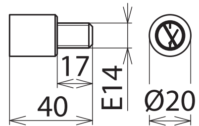
Maßbild SE E14
