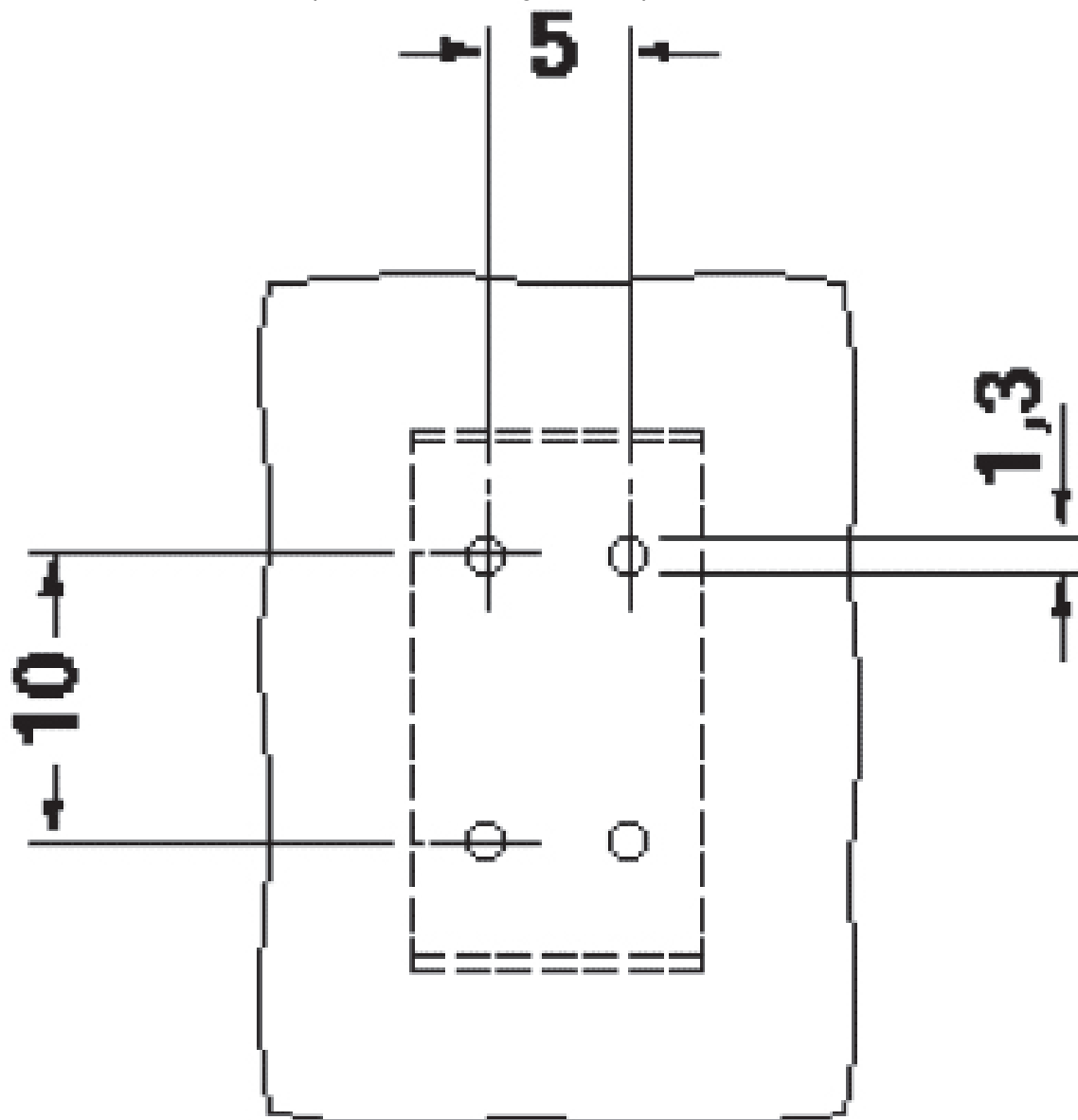
Esquema de taladros/geometría pads soldadura
