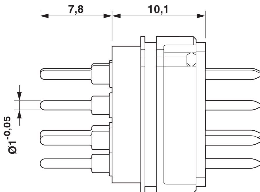
Dessin coté
