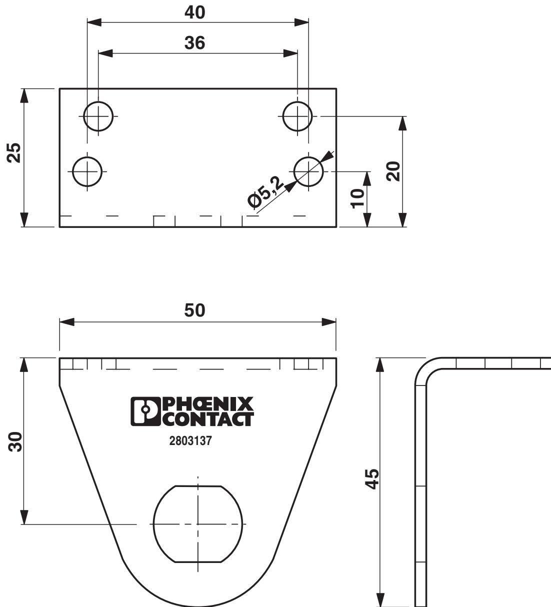
Maßzeichnung
