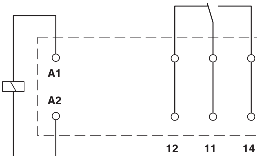
Schaltplan
