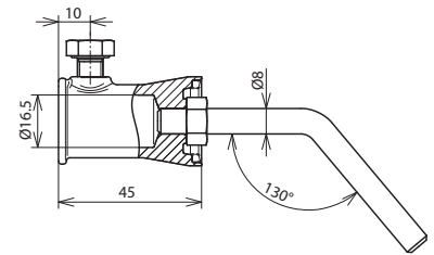
Maßbild BA130 RD8 BB16 V2A ZG
